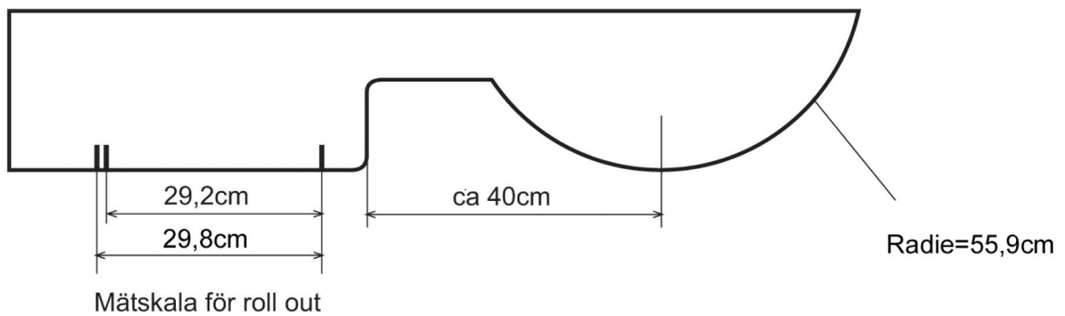
Figur 2. Kontrollmall för mätning av roll out
