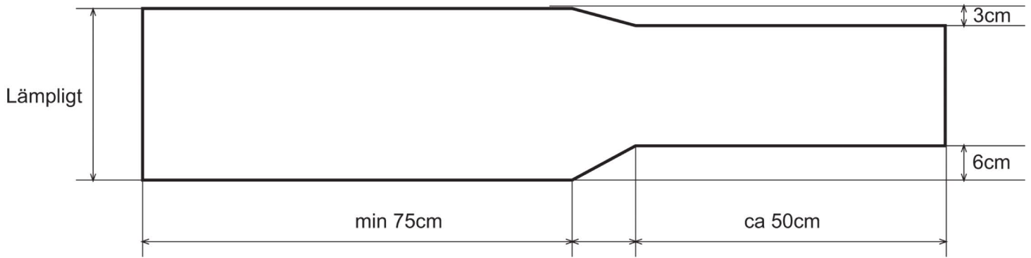
Figur 1. Kontrollmall för höjdmätning av fotoceller i startområdet
