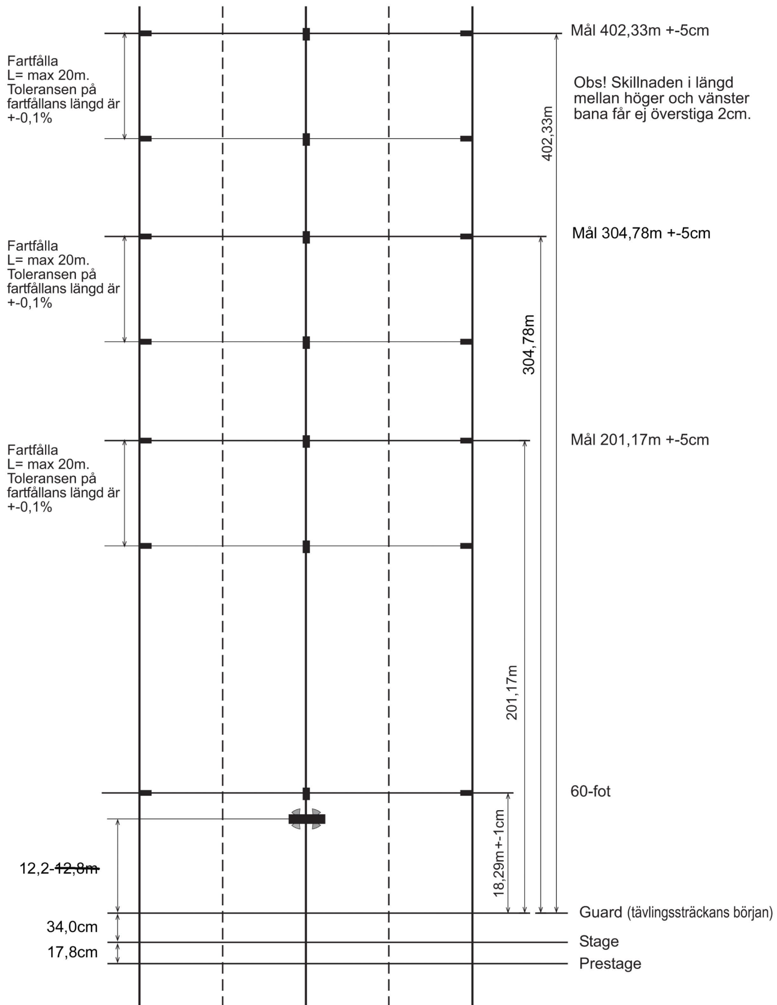
Figur 5. Banmått
